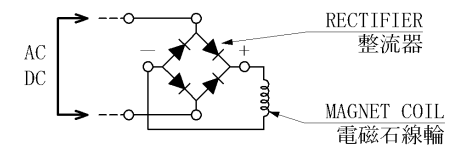
CONNECTION DIAGRAM 結線図
